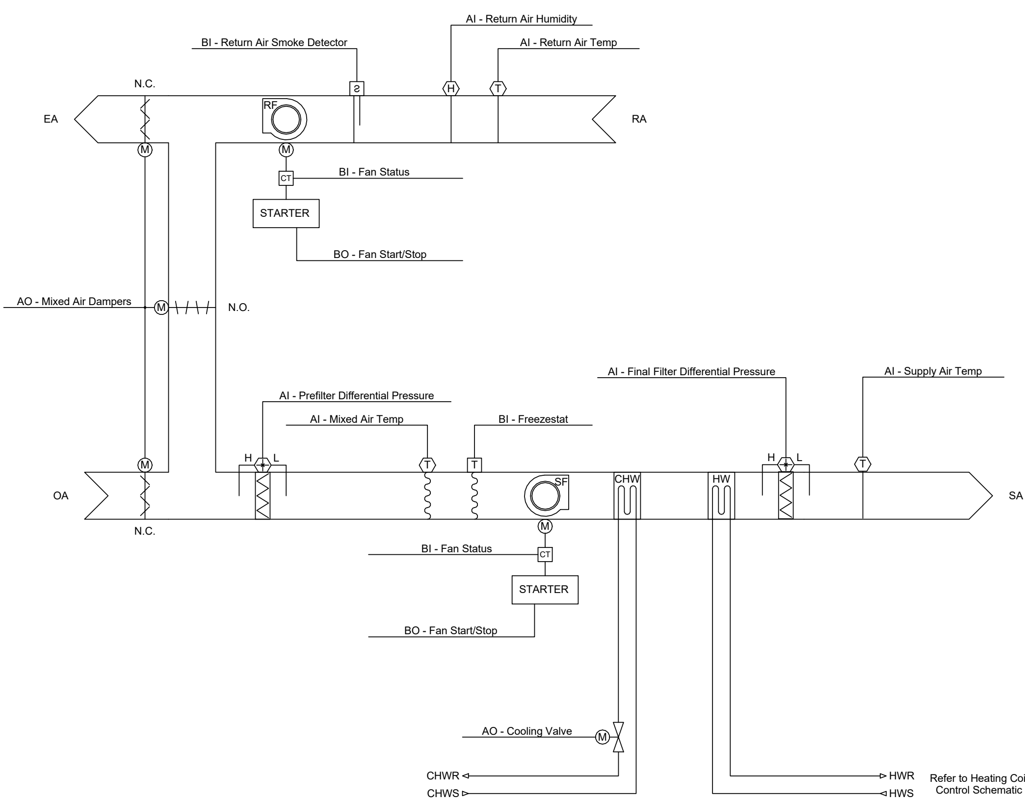
AHU-1 (AUDITORIUM) CONTROL SCHEMATIC (CONSTANT FLOW) SCALE: N.T.S.
