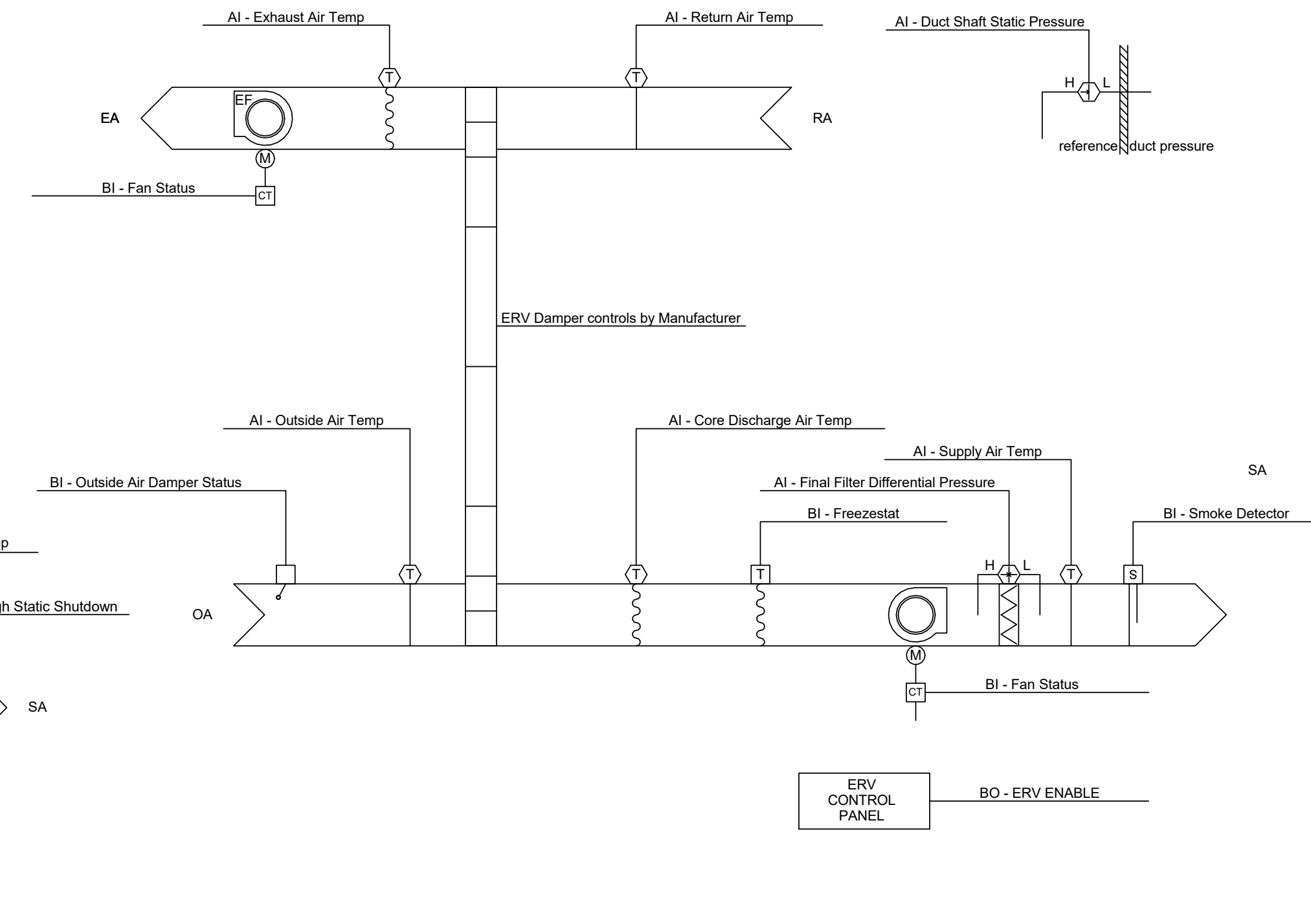
ERV-1 AND ERV-2 CONTROL SCHEMATIC SCALE: N.T.S.
